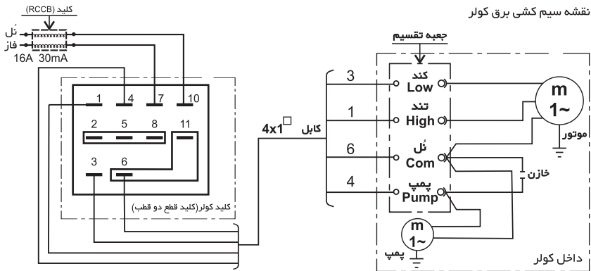
نقشه سیم کشی برق کولر
