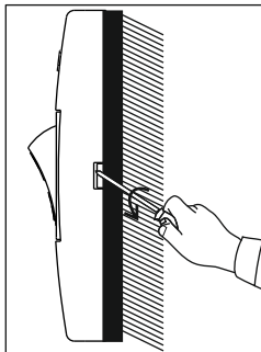
نصب قاب کلید روی صفحه کلید
